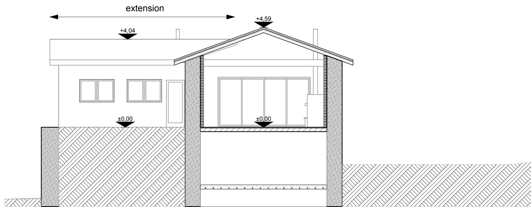
coupe/façade 4 3
