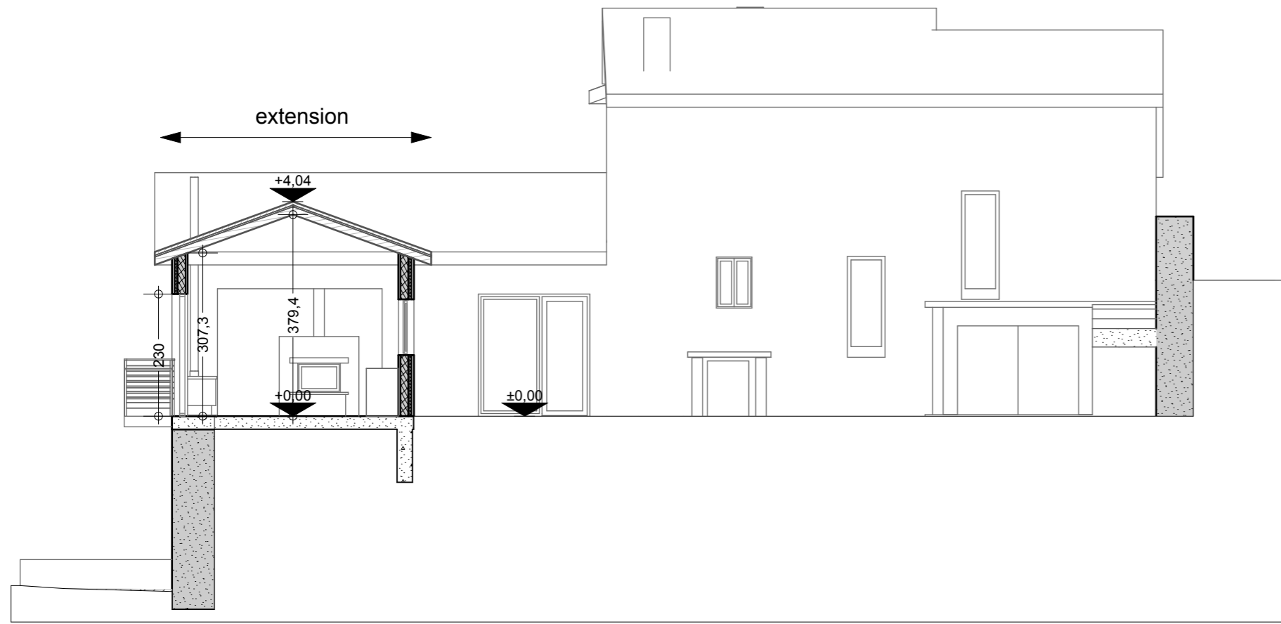
coupe 3
