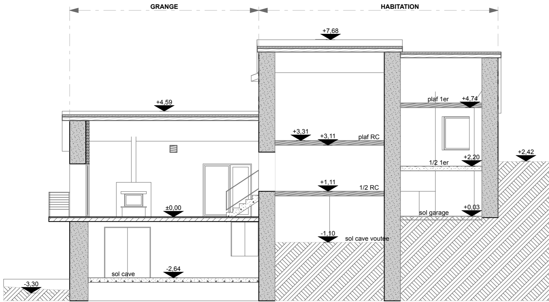
coupe 1
